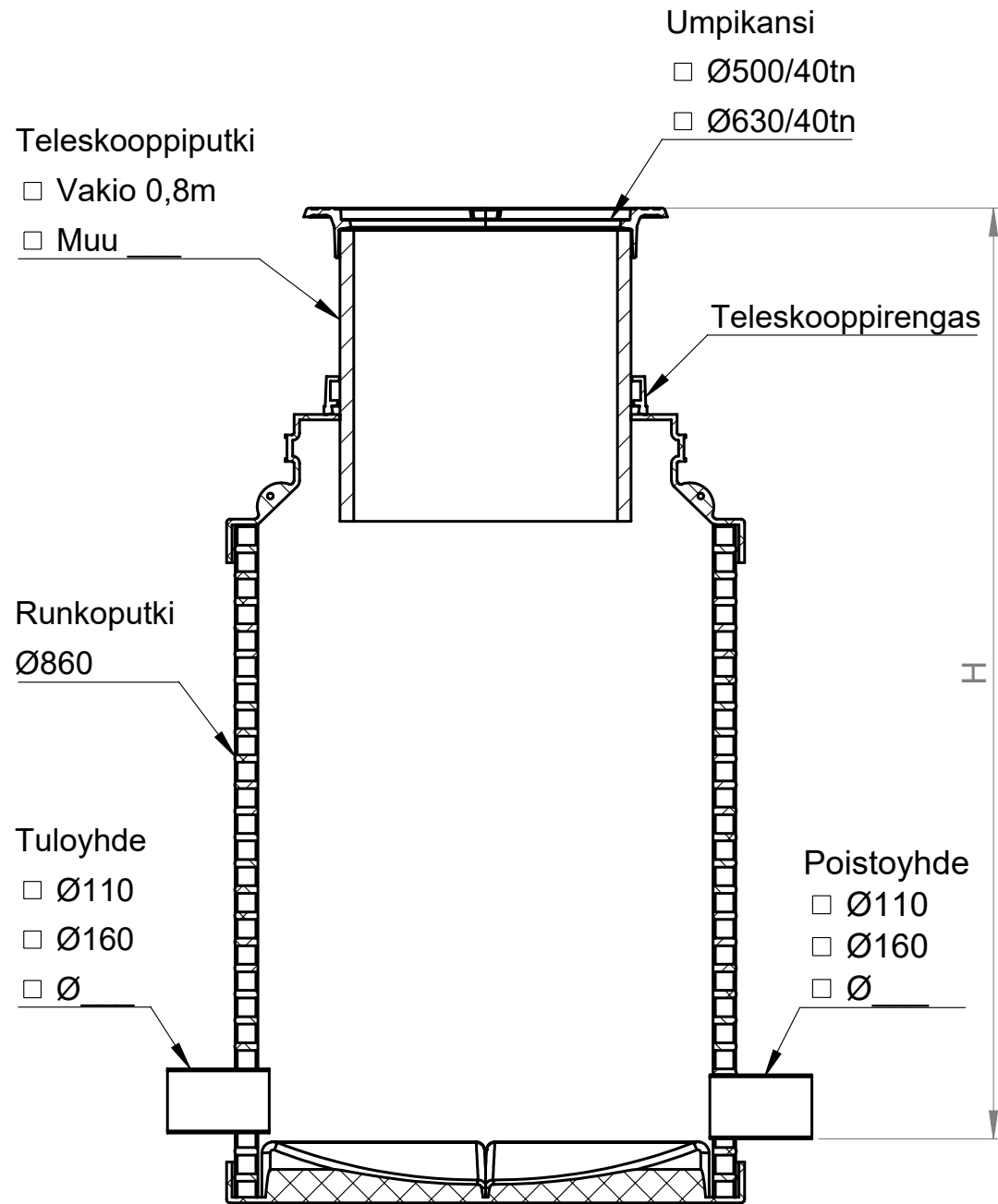
SECTION A-A SCALE 1 : 12
