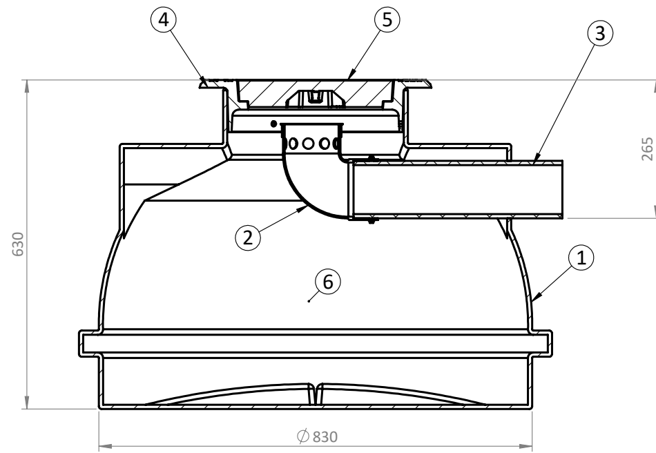
SECTION A-A
