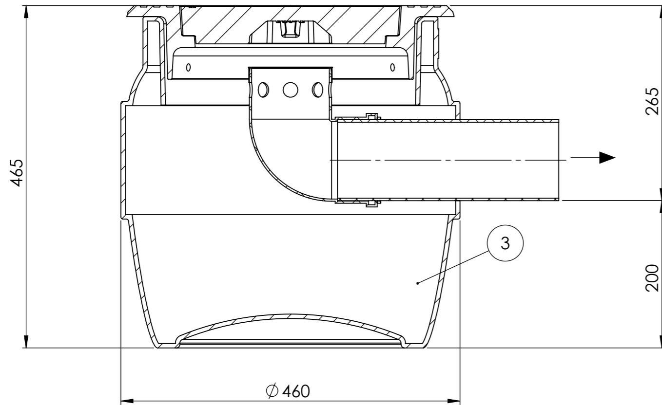
SECTION A-A
