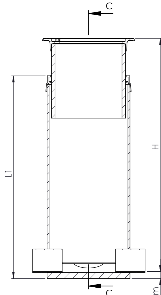
SECTION A-A SCALE 1 : 13
